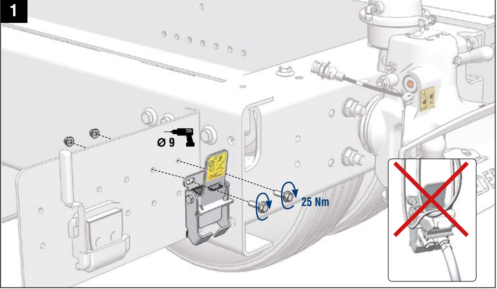
(Duomatic-) Druckluftschlauchhalter montieren. | Assemble the (Duomatic-) compressed air hose holder.
